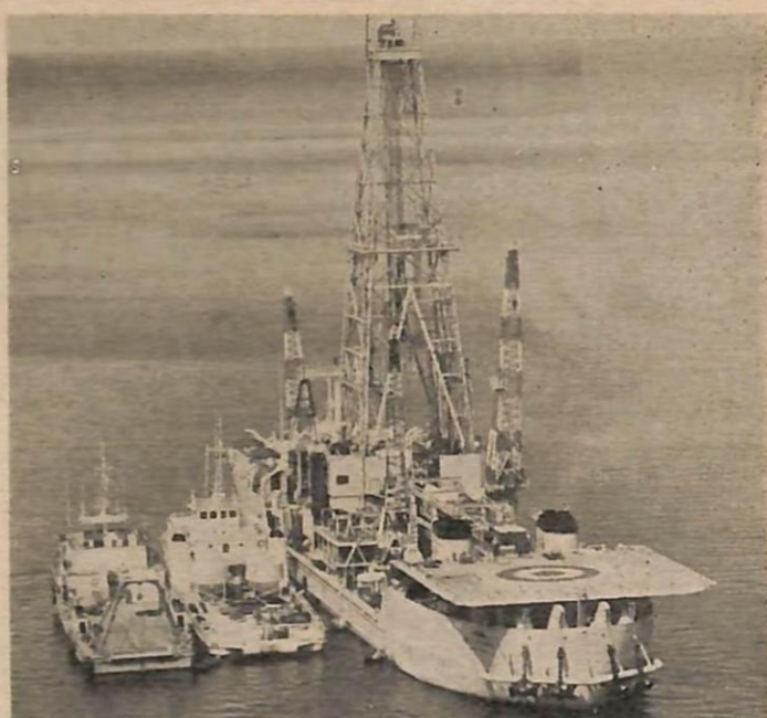
KAPAL pengorek yang terbesar di-dunia — SEDCO 445 (gambar di-atas) telah mula menjalankan pengorekan di-perayeran Brunei.
