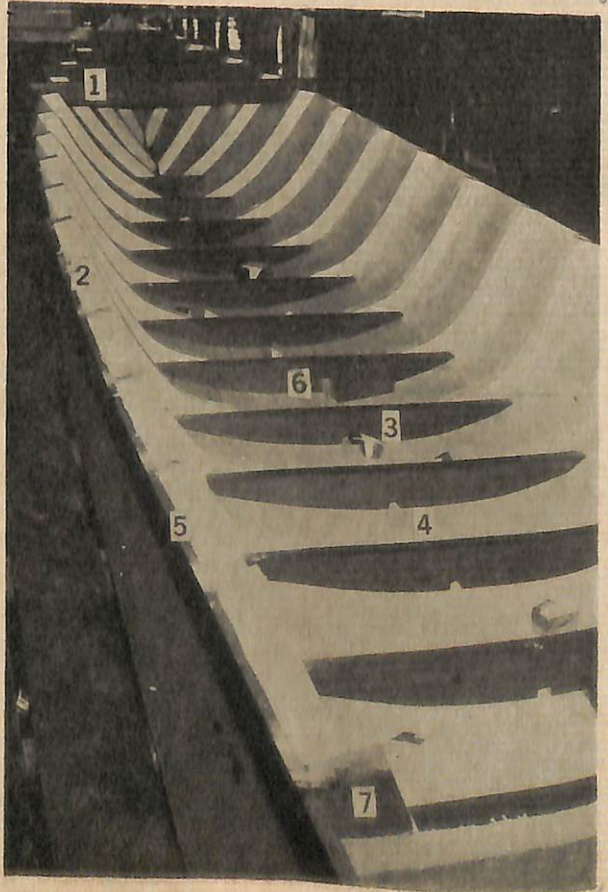
Bahagian charok sa-buah perahu yang hampir siap. Kelima2 kayu melintang itu di-namakan "sangkar".
