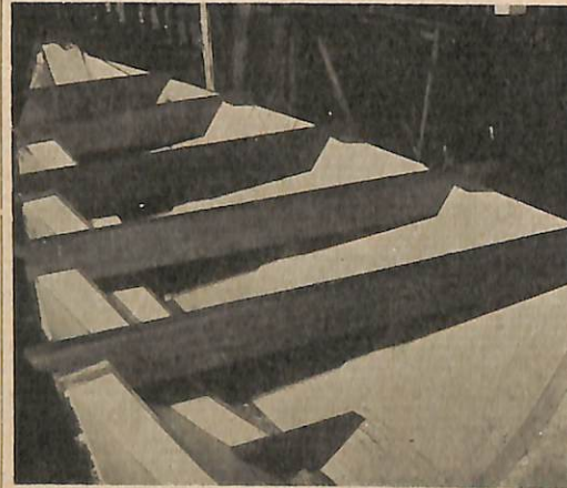
Bahagian charok sa-buah perahu yang hampir siap. Kelima2 kayu melintang itu di-namakan "sangkar".
