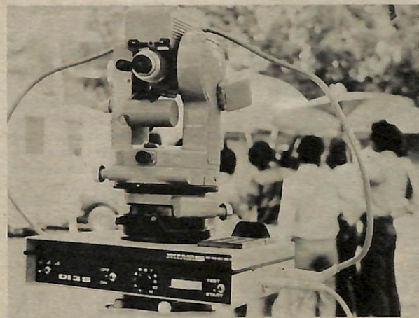
GAMBAR di-atas ini ia-lah Distomat, ia-itu alat pengukur jarak elektronik yang boleh menghasilkan satu2 penyukat-an jarak dalam masa yang pendek dan boleh menyukat sa-jauh 1000 meter.
