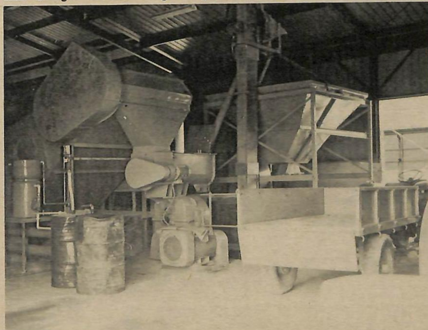
JENTERA2 moden bagi mengisar padi memainkan peranan yang penting dalam mempercepatkan kerja2 memproses padi. Projek ini di-jalankan bertempat di-Jerudong.
