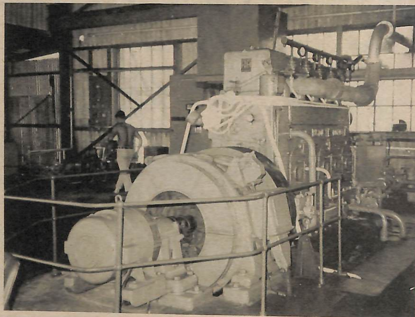
INI ia-lah salah sa-buah generator yang telah membekalkan letrik kepada penduduk2 Pekan Bangar dan beberapa buah mukim lagi. Bekalan letrik bagi daerah ini akan di-tambah daripada yang ada sekarang kepada 1MW.
