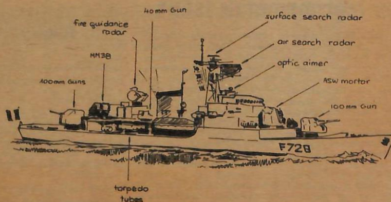
KEBAWAH DYTM mendengar taklimat mengenai fungsi dan keupayaan kapal tersebut oleh Kapten Olhagaray. GAMBAR rajah menunjukkan kedudukan senjata-senjata dan peralatan-peralatan yang digunakan oleh kapal Doudart de Lagree.
