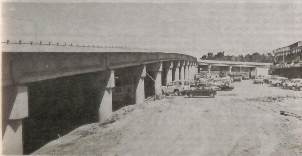
JEJATAS menyeberangi sungai dan Jalan Gadong ini berukuran 522 meter, ianya nanti memberikan kemudahan lalu lintas di Kawasan Jalan Gadong (atas). SATU selekoh yang terdapat pada jejatas di kawasan Gadong (kanan).
