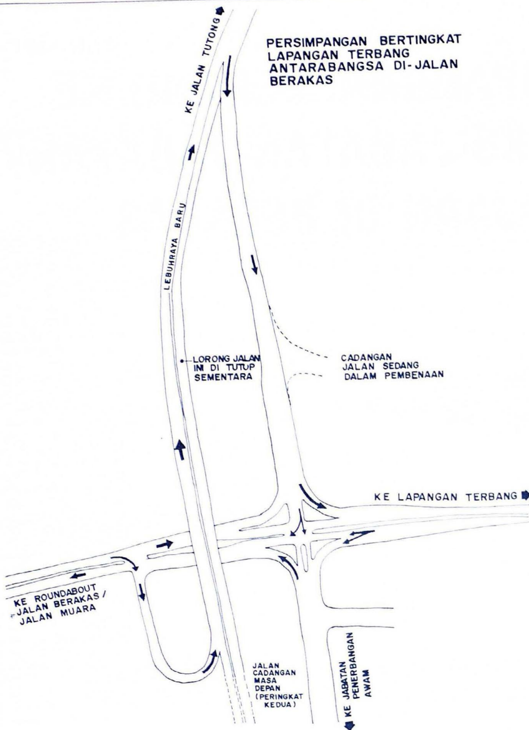
PERSIMPANGAN bertingkat (flyover) di Lapangan Terbang Antarabangsa Berakas sepanjang 180 meter. Flyover ini akan menghubungkan Batu 6 Jalan Muara terus ke Jalan Sungai Akar apabila projek peringkat kedua dilaksanakan nanti.
