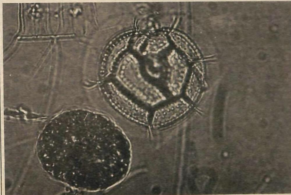
GAMBAR mikroskop 'Pyrodinium Bahamese' yang telah menyebabkan air kemerah-merahan di Negara Brunei Darussalam.
