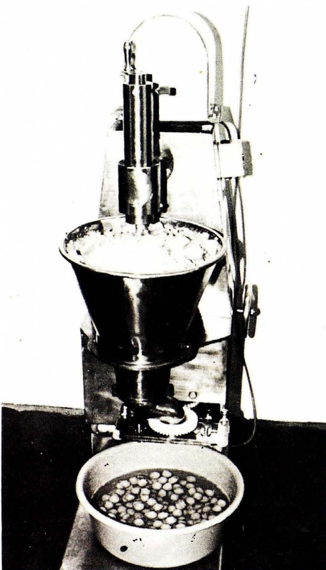
MESIN membuat bebola ikan yang terdapat di Kompleks Pendaratan Ikan di Muara dijangka akan dapat menambahkan 'added value products'.
