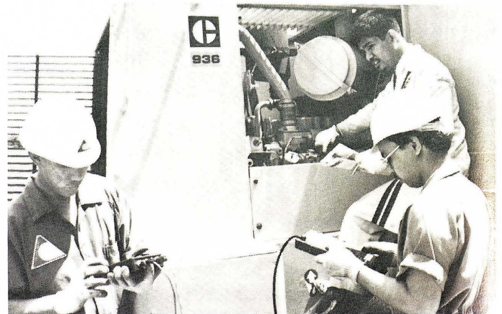
TIGA daripada pelatih di Pusat Latihan Mekanik sedang melakukan kerja-kerja pembaikan dan pemeliharaan jentera berat di pusat berkenaan.
